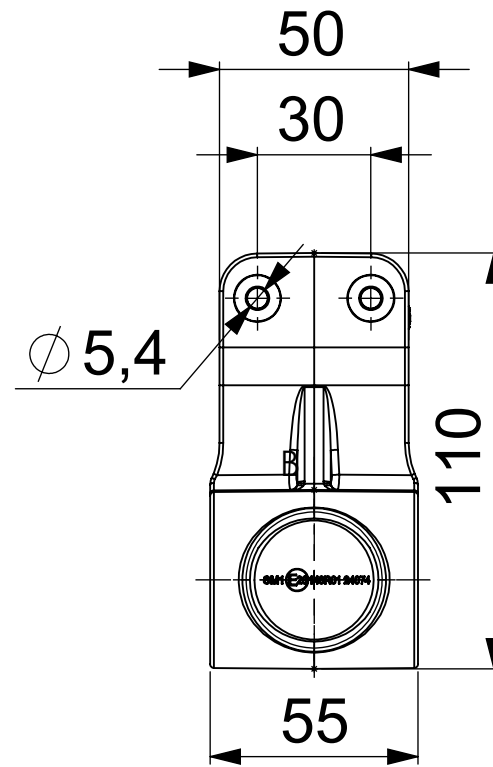
SZCZEGÓŁ B
