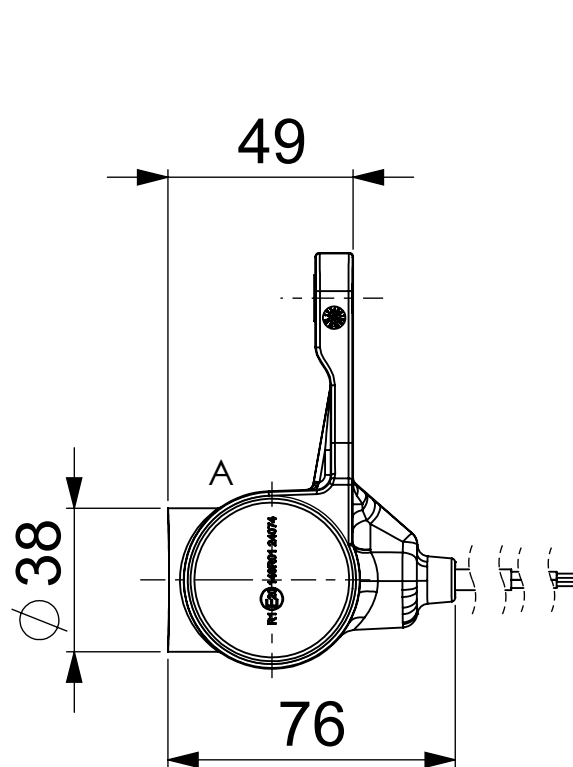
SZCZEGÓŁ A
